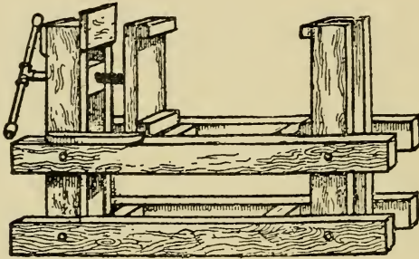
Fig. 31.—HOPKINS' HIVE CRAMP.
