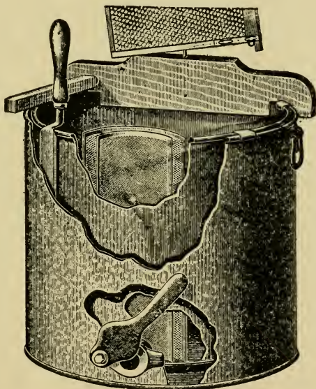
Fig. 46.—ROOT CAPPINGS-MELTER.
