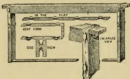
Fig. 33.—METAL-SPACED FRAME.
